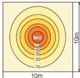
照度分布図 (単位:lx 取付高さ:2.23m)
